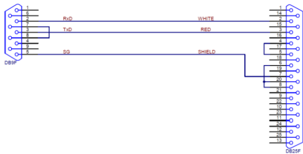
Fig. 2: DB9F-DB25F
